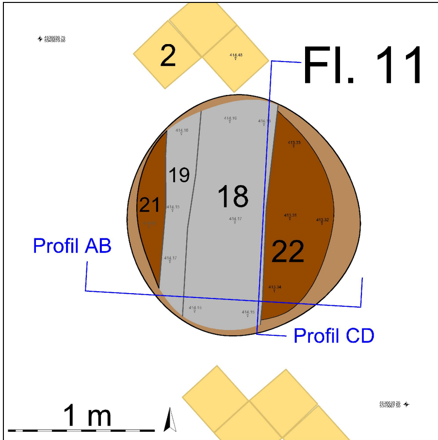
Schnitt 11: Planum 0 und 2 und 5. M. 1:25.
