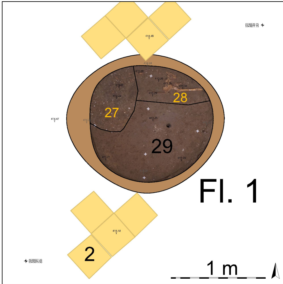
Schnitt 1: Planum 0 und 5. M. 1:25.
