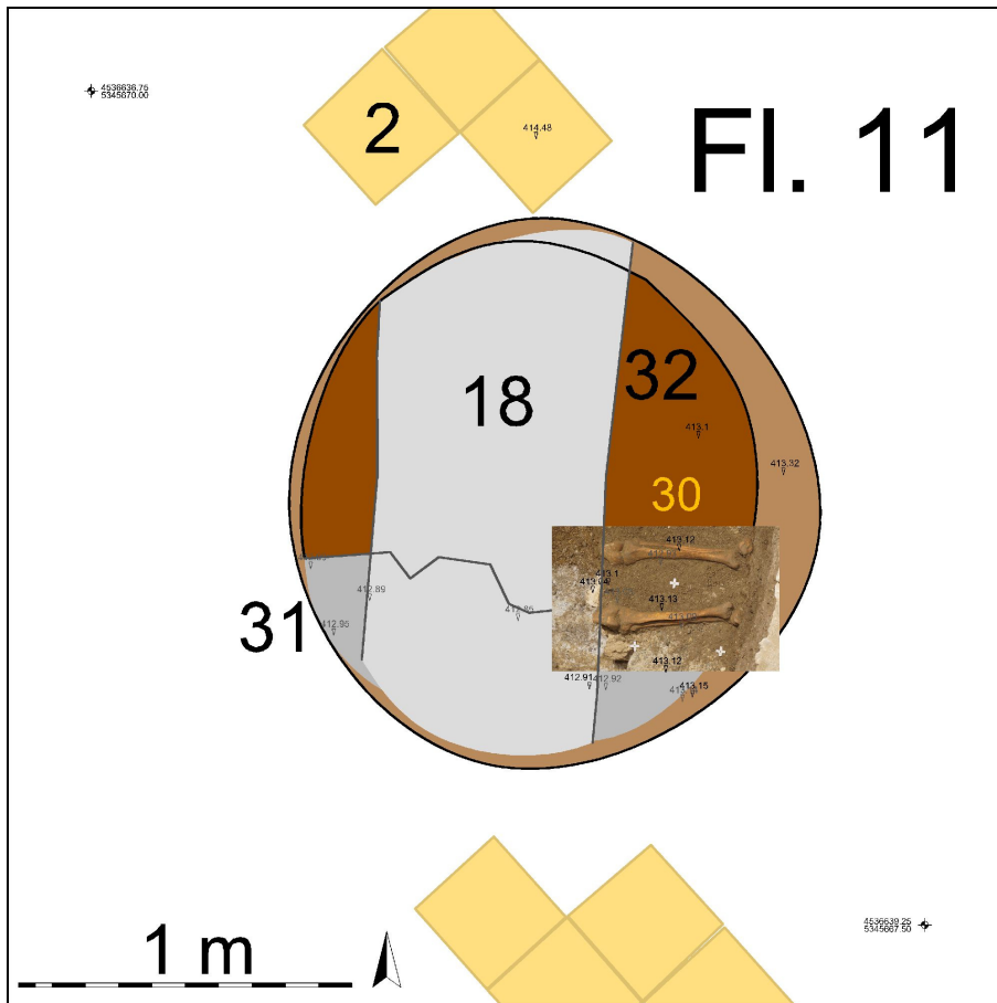
Schnitt 11: Planum 0 und 2 und 6 und 7. M. 1:25.
